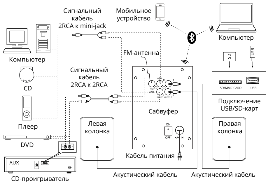
Рис. 4. Схема подключения
