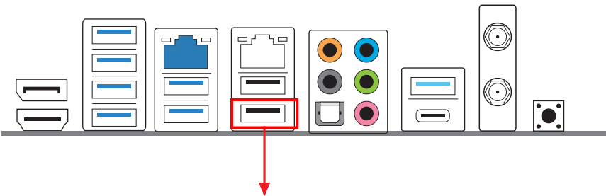
USB-BIOS-Flashback-Port
