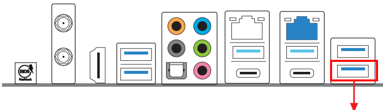
USB-BIOS-Flashback-Port
